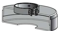
Ochranný kryt typ 41
