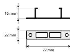
Přichytka nosníku k podkladu (N1)
