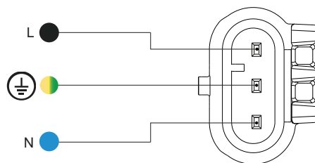
Síťová zástrčka
