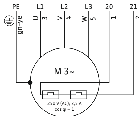
Fig. 5: Schéma zapojení 3~ motoru
