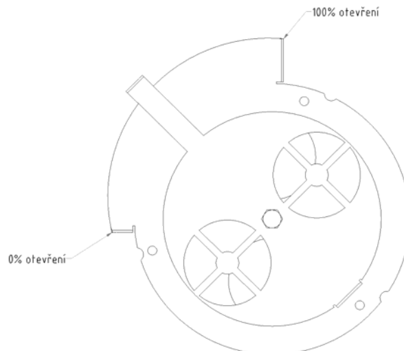
Obr. č. 12 Škrťící klapka ventilátoru
