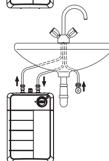
EO 15 P s montáží pod umývadlo – beztlaková přípojka
