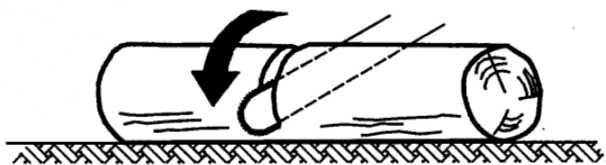
Ilustracija BB.104-Deblo podprto po celotni dolžini
