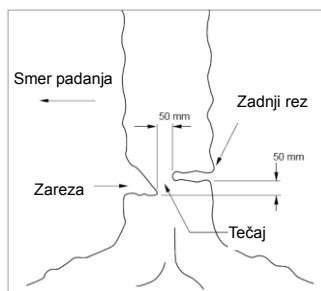
Ilustracija BB.102-Opis podiranja dreves: spodrezovanje
