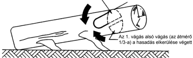
BB.105 ábra Egyik végénél alátámasztott fatörzs
