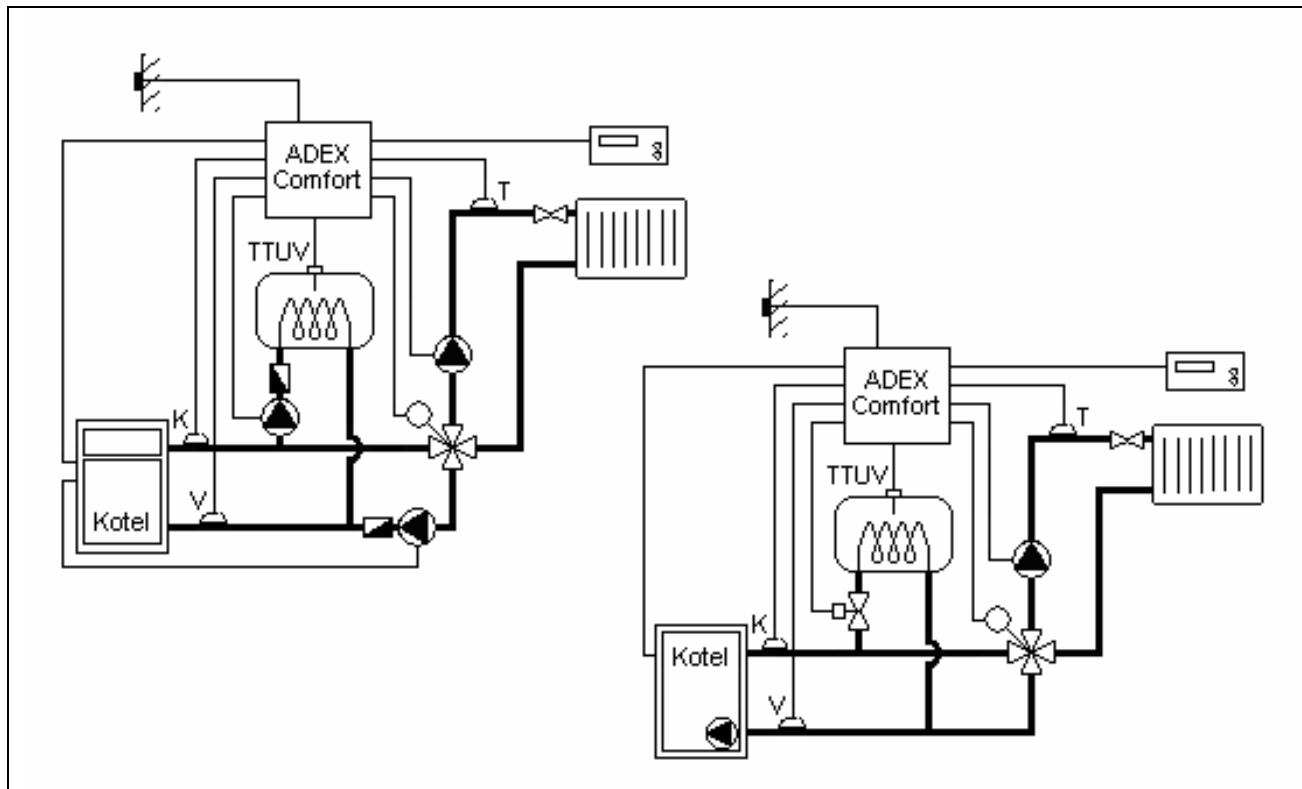
Obr. 2 Funkční schéma zapojení pro Systém 1
