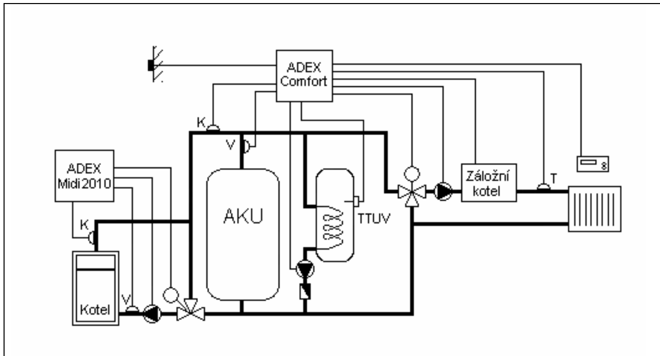
Obr. 16 Funkční schéma zapojení pro Systém 8
