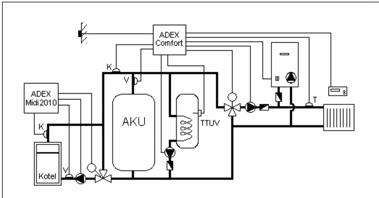
Obr. 14 Funkční schéma zapojení pro Systém 7
