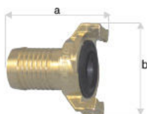
GEKA PLUS TRN - kód 30180 GEKA PLUS SS TRN - kód 30186
