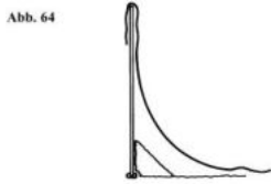
FALSCH! LASSEN SIE KEINE LÖCKE ZWISCHEN DER FOLIE UND DER WÖLBUNG. DADURCH WIRD AUF DIE FOLIE EIN DRUCK NACH UNTEN AUSGEÜBT. BERICHTIGEN SIE DIESEN ZUSTAND, FALLS ER EINTRIT.
