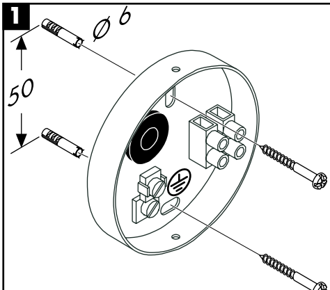
QT 20 HalogenA 230 V / E14 / max. 40 Watt
