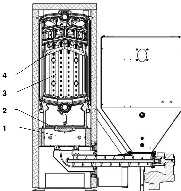
Obr. č. 7 Řez kotlem
