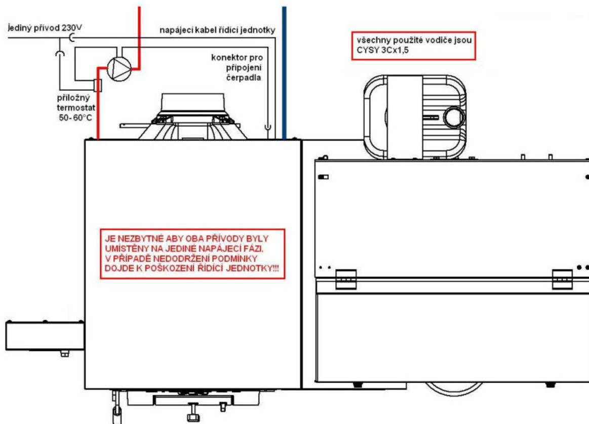
Obr. č. 5 Zapojení oběhového čerpadla kotle
