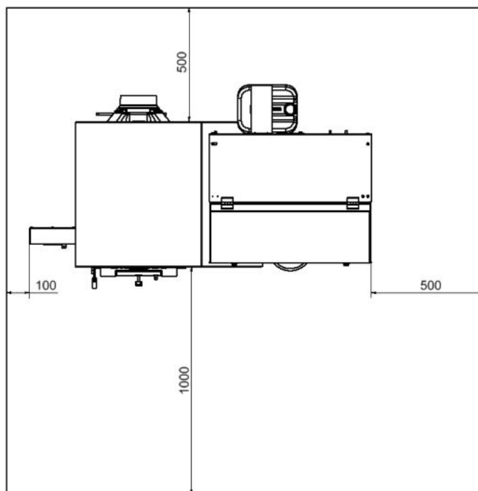
Obr. č. 3 Umístění kotle v kotelně
