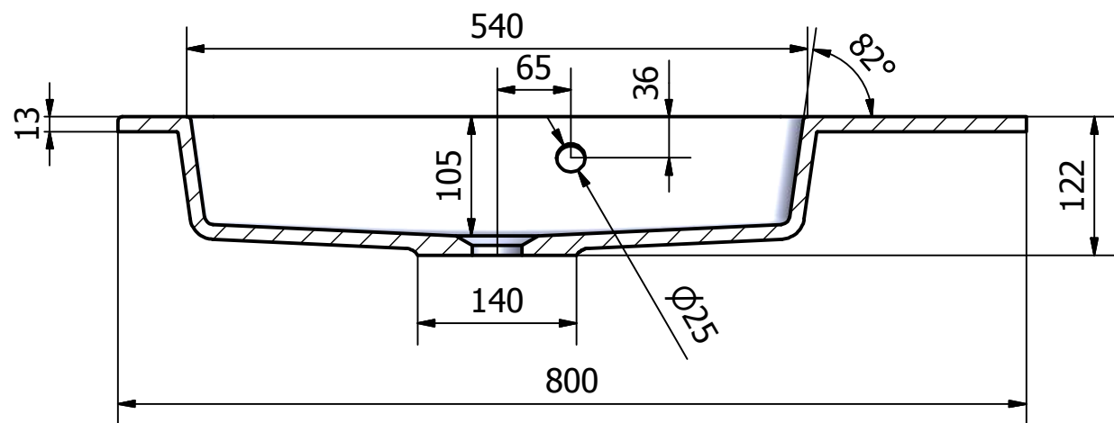
A-A (1 : 6)
