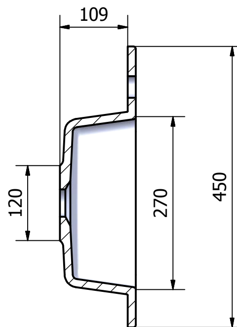
B-B (1 : 6)
