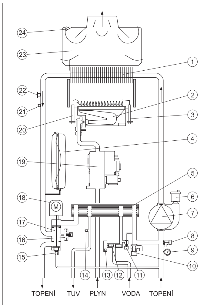
LEGENDA: Příklad kotle s odtahem spalin do komína a ohřevem TUV v deskovém výměníku
