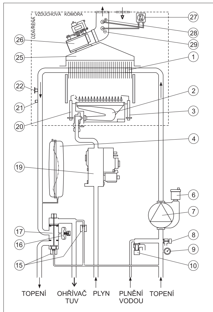
LEGENDA: Příklad kotle s odtahem spalin ventilátorem a vestavěným 3-cest.ventilem pro ohřev TUV v zásobníku
