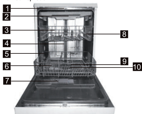
Pohled zepředu
