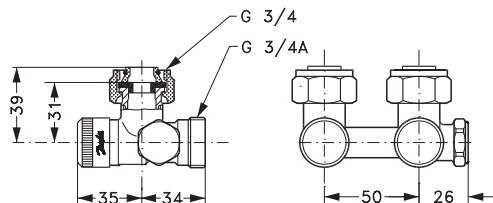
RLV-K rohové s přípojovacím hrdlem na topné těleso G3/4
