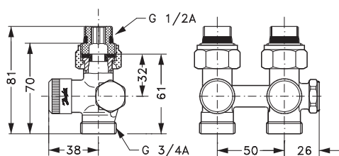
RLV-K přímé s přípojovacím hrdlem na topné těleso G3/4
