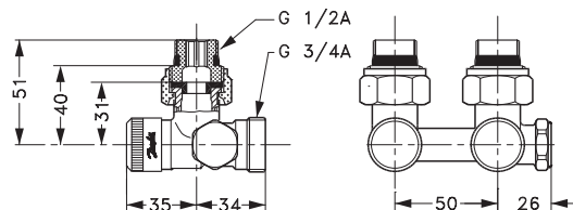
RLV-K rohové s přípojovacím hrdlem na topné těleso G1/2 A
