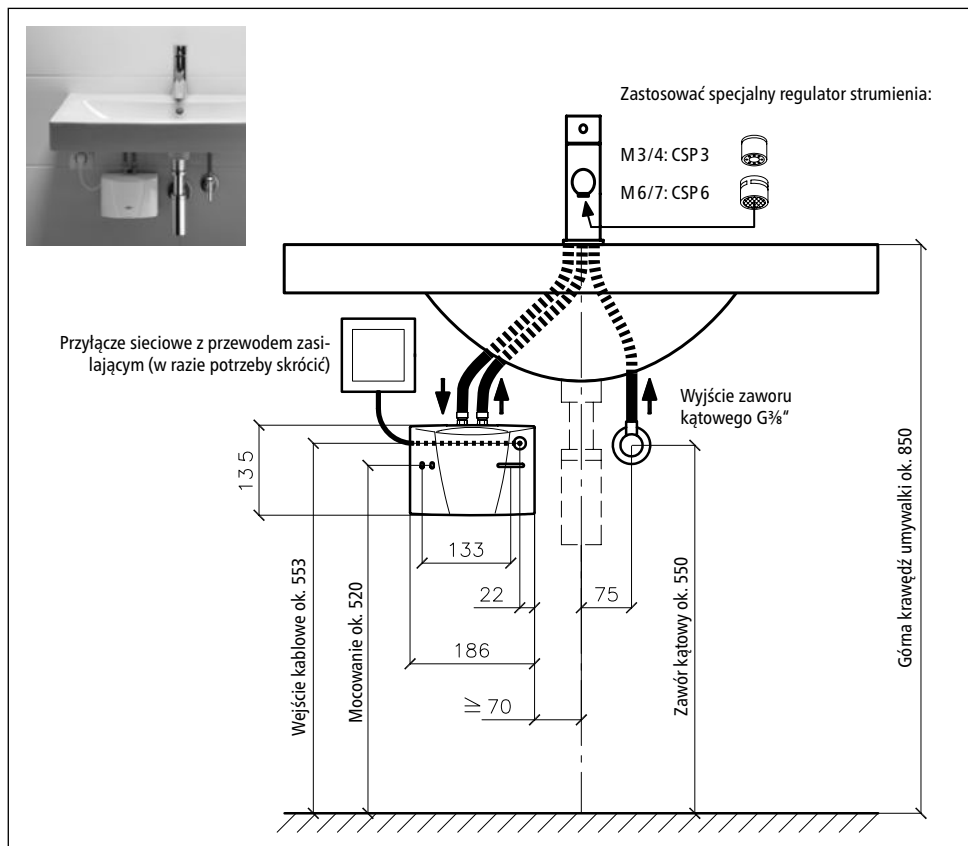
Rys. 3: »Bezcisnieniowa (otwarta) instalacja z armaturą do bezciśnieniowych urządzeń do wody ciepłej« (wymiały w mm)
