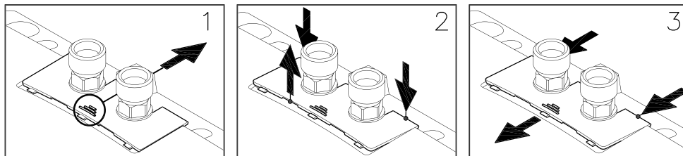
Kuva 8: »Levyn irrottaminen«
