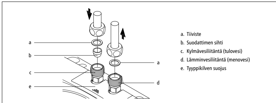
Kuva 5: "Vesijohtojen kytkeminen"
