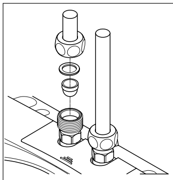
Kuva 11: "Siivilän vaihtaminen"
