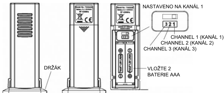
SNÍMAČ VENKOVNÍ TEPLoty
