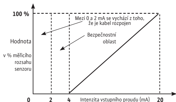
Signál senzoru 4–20 mA
