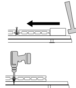
Montáž posledního prkna
