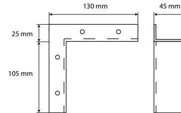
fixační úhelník vnější (N3)
