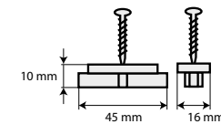
Příchytka terasového prkna k nosníku (P1) s ocelovým šroubem s černým šroubem
