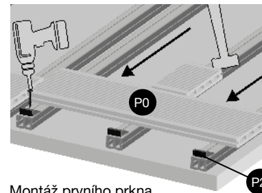
Montáž prvního prkna
