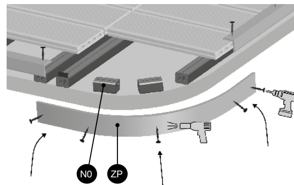
Zakončovací lišta plochá (ZP) 0,9 / 9 / 200 cm
