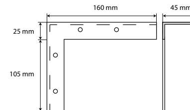
fixační úhelník vnitřní (N2)
