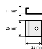
Startovací příchytka terasového prkna k nosníku (P2)
