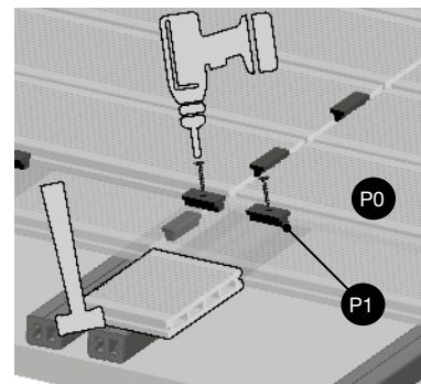
Montáž prvního prkna
