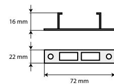
Příchytka nosníku k podkladu (N1)
