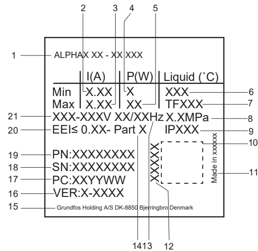
Typový štítek
