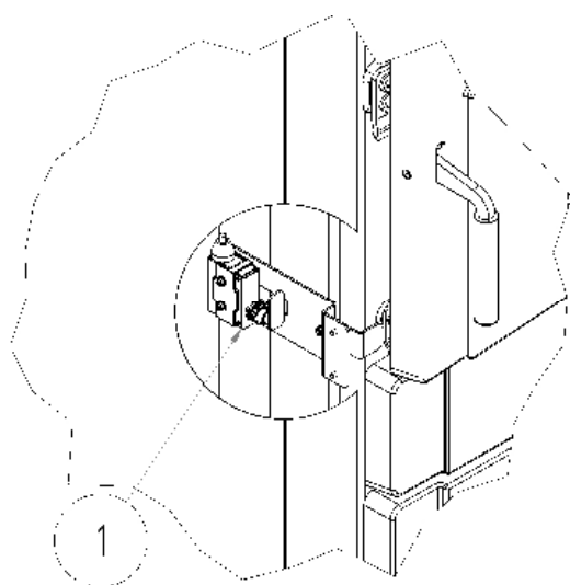
1. Koncový spínač
