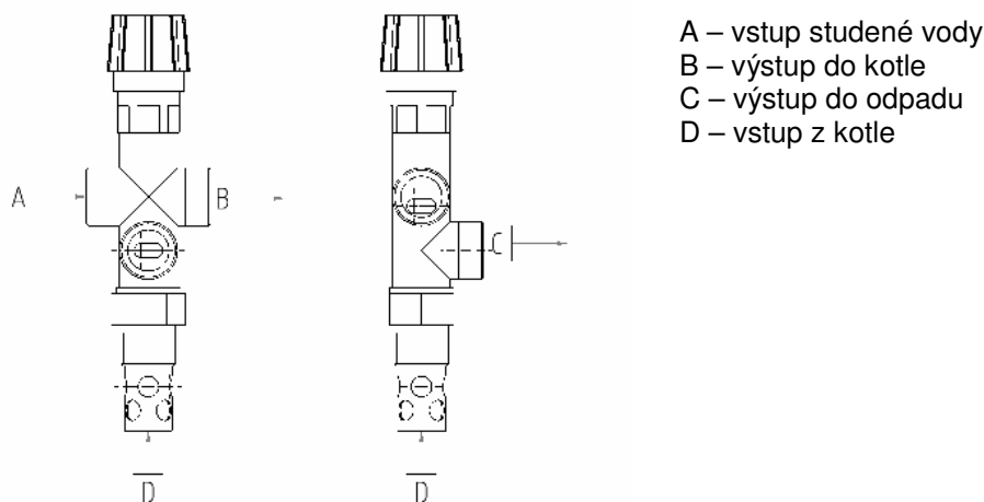
Obr. č. 23 Dvoucestný bezpečnostní ventil DVB 1 – 02
