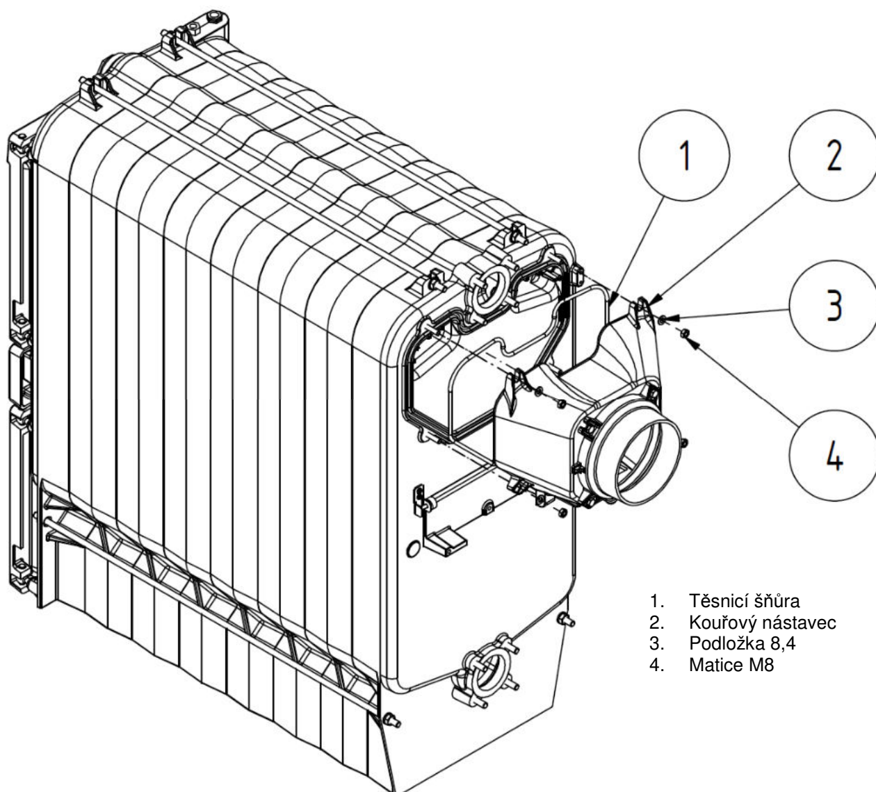
Obr. č. 7 Montáž kouřového nástavce
