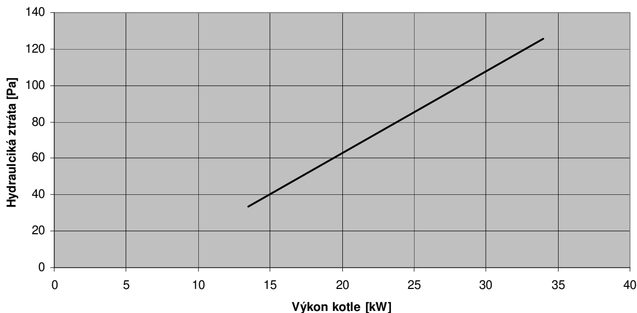
Obr. č. 1 Hydraulická ztráta kotlového tělesa
