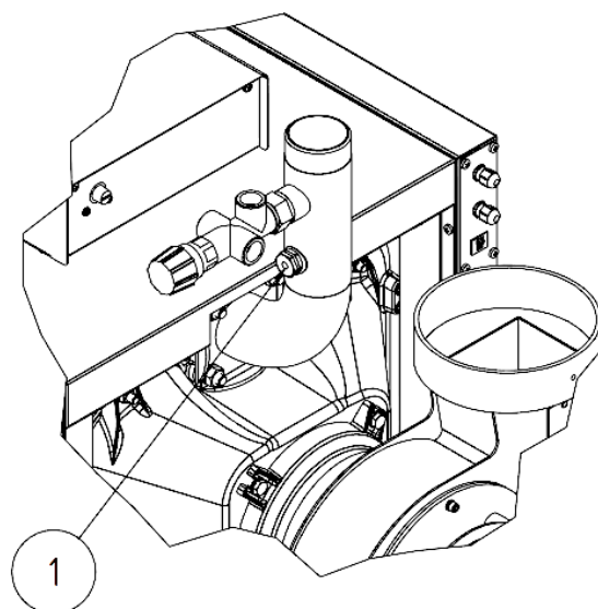
Obr. č. 15 Umístění jímky čidla ÚT
