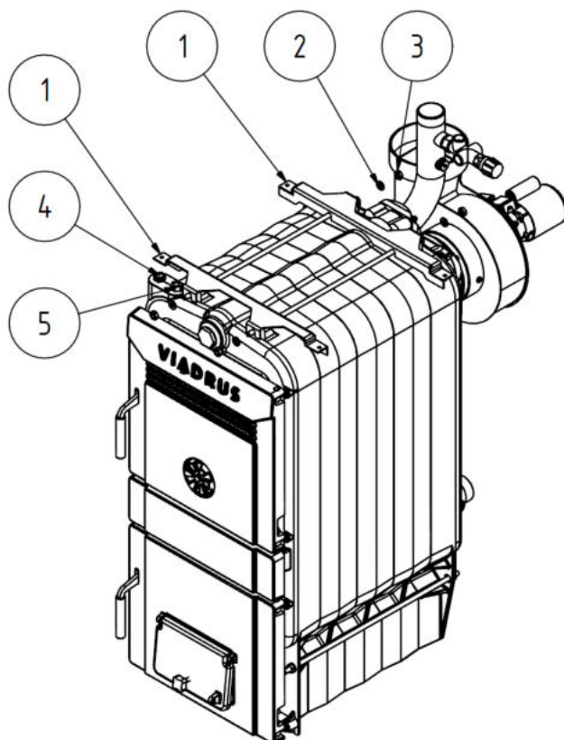
Obr. č. 11 Montáž konzol pláště
