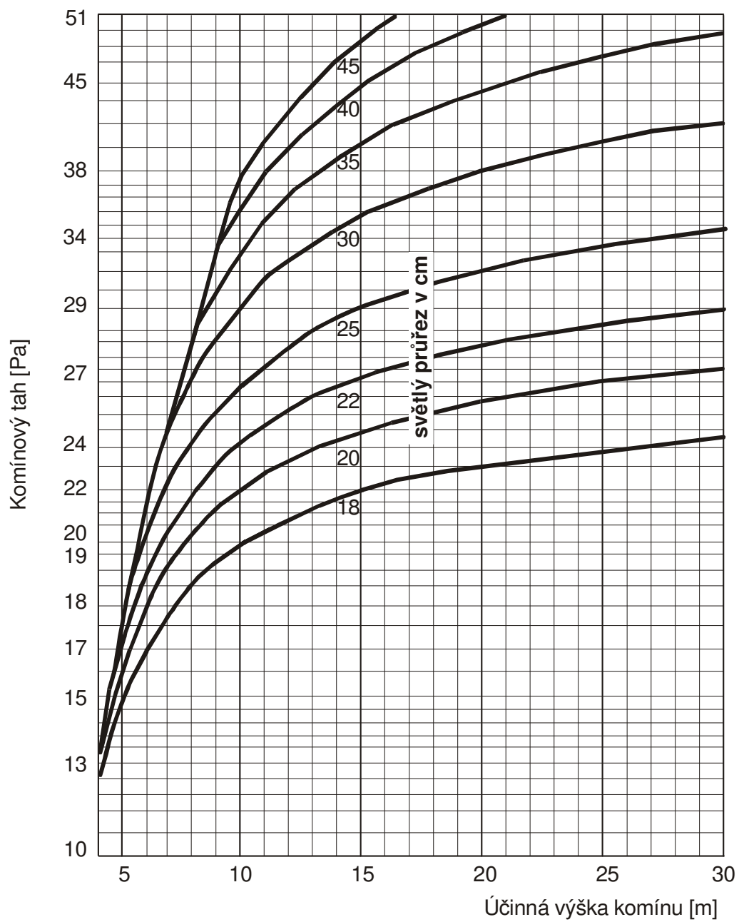
Obr. č. 2 Stanovení průměru komínu
