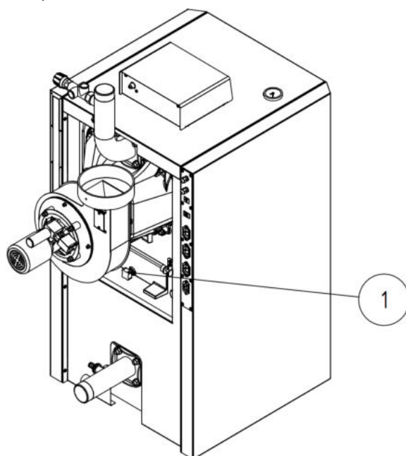
Obr. č. 16 Šroub dusivky
