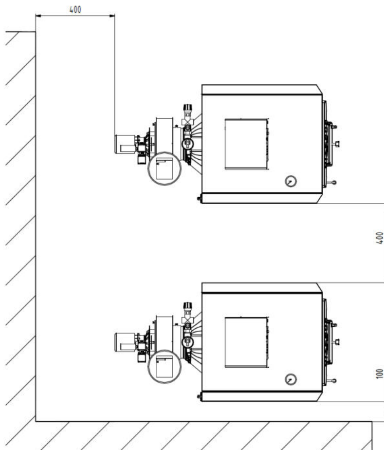
Obr. č. 6 Umístění kotlů v kotelně
