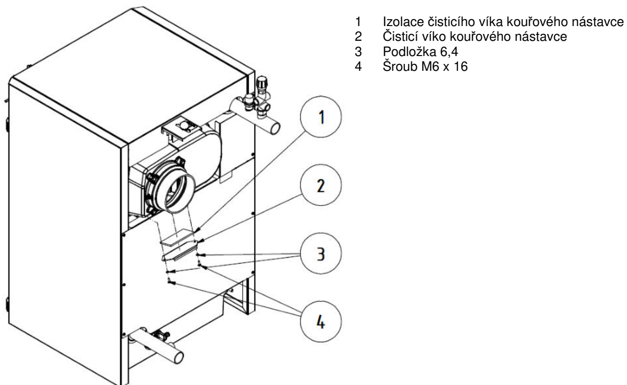
Obr. č. 21 Čištění kouřového nástavce
