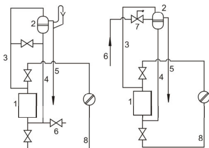
Obr. č. 17 Příklady zapojení otevřených expanzních nádob
