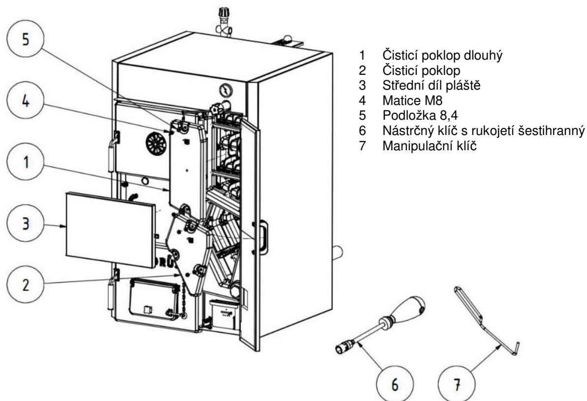
Obr. č. 20 Demontáž čisticího poklopu
