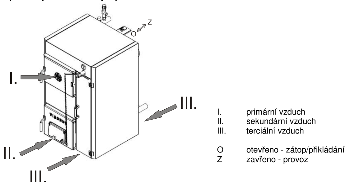
Obr. č. 18 Přívod vzduchů do kotle
