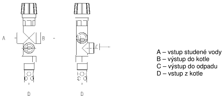
Obr. č. 15 Dvoucestný bezpečnostní ventil DBV 1 – 02
