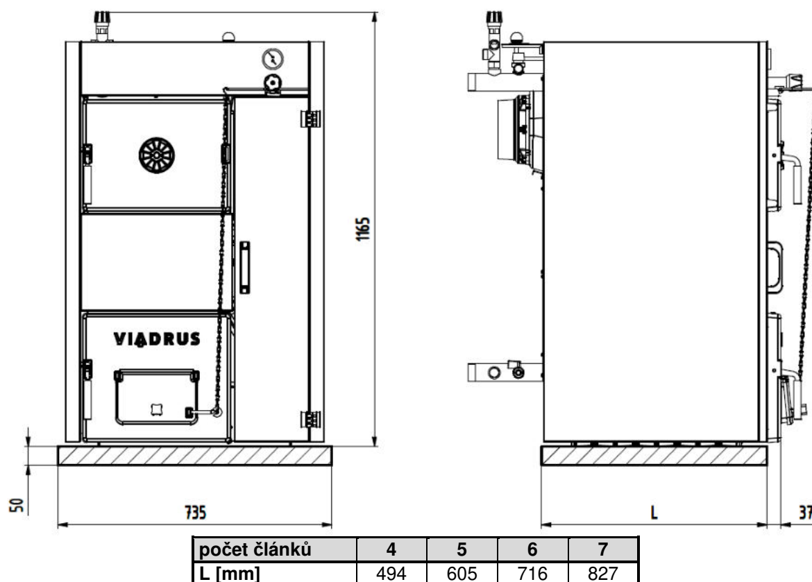
Obr. č. 4 Rozměry podezdívky
