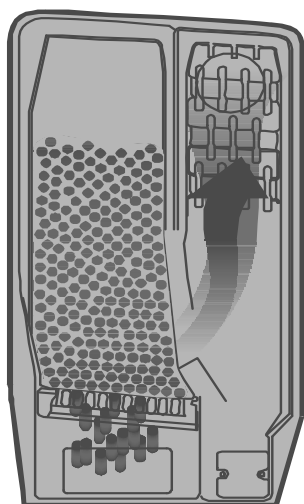
Obr. č. 19 Schéma průchodu spalin kotlem
