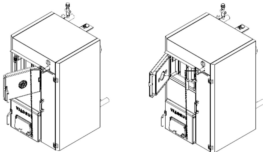
Obr. č. 5 Varianty otevírání příkládacích dvířek
