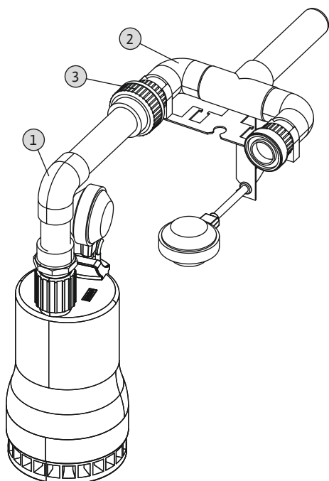
Fig. 13: Demontáž čerpadel
