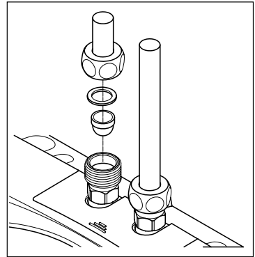
Obr. 12: «Výměna vložky filtru»
