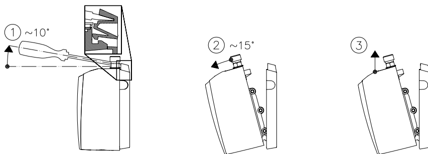
Rys. 14: »Zdejmowanie urządzenia z uchwytu ściennego«
