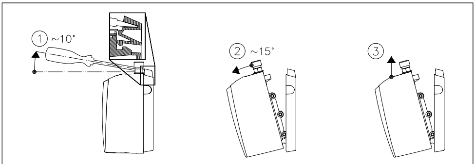
Abb. 14: »Abnehmen des Gerätes aus dem Wandhalter«
