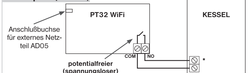
Schaltplan (Abb. 4)
