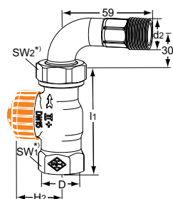
Durchgang mit Bogenverschraubung
