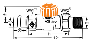
Durchgang mit Viega Pressanschluss 15 mm
