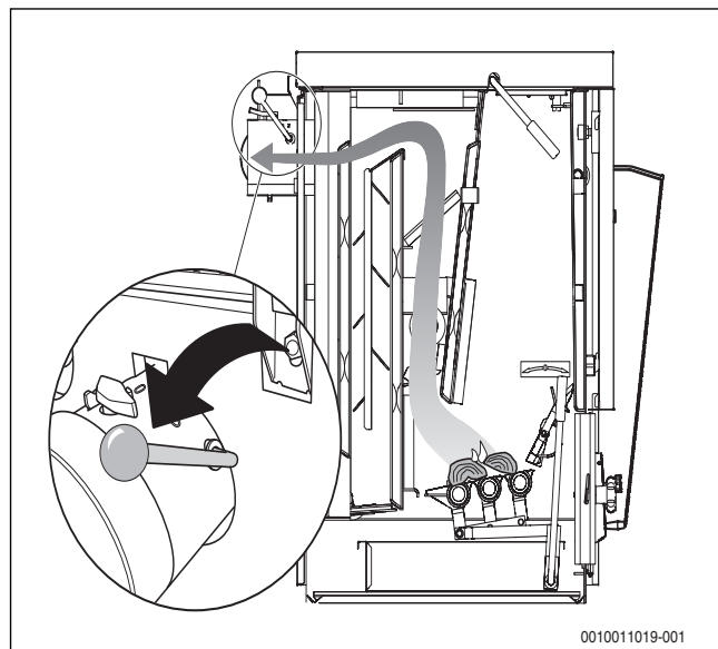
Obr. 3 Roztápěcí klapka v roztápěcí poloze
