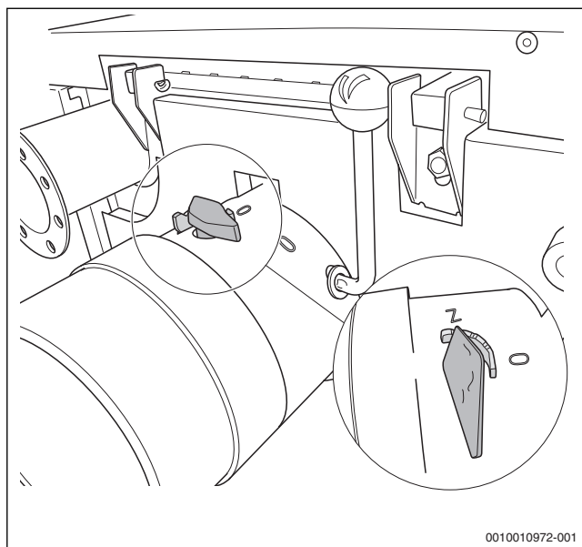
Obr. 5 Nastavení spalínové klapky
