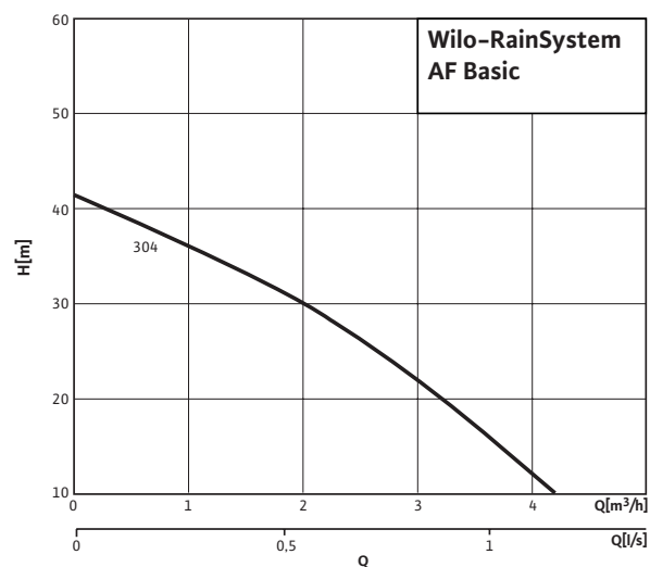
Wilo-RainSystem AF Basic
