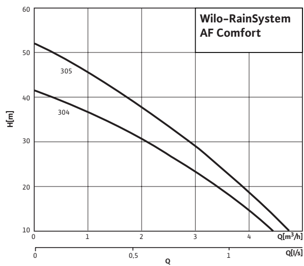
Wilo-RainSystem AF Comfort
