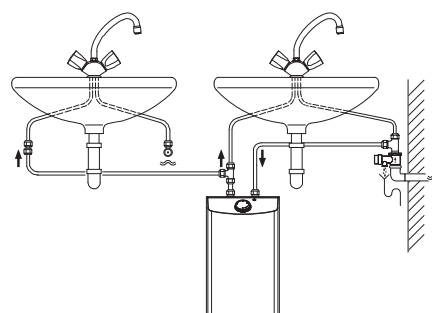
EO 10 P s montáží pod umývadlo
