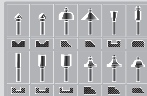
Obr. 1, tvar profilů v závislosti na použité tvarové frézě
