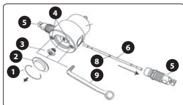
Obr.5, výměna jehly
