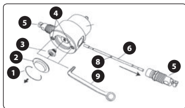
Abb. 5, Austausch der Nadel Fig. 5, Punch replacement
