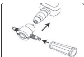
Obr.4, instalace rukoveti a uchytení do vrtáčky
