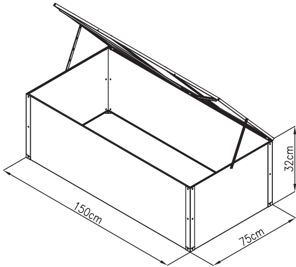
Dimensions \ Abmessungen \ Rozměry \ Rozmery \ Méretek \ Wymiary
