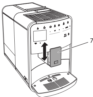
Fig. 12: Højdejusterbart udløb
