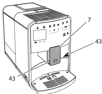
Abb. 23: Milcheinheit ausbauen, 1
