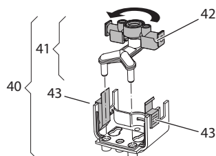
Bild 19: Vrida inloppet, 2
