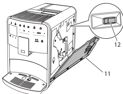
Kuva 17: Jauhatusasteen säätäminen
