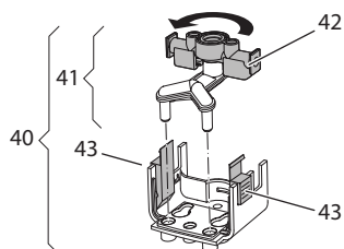
Kuva 19: Syöttöyksikön kääntäminen, 2
