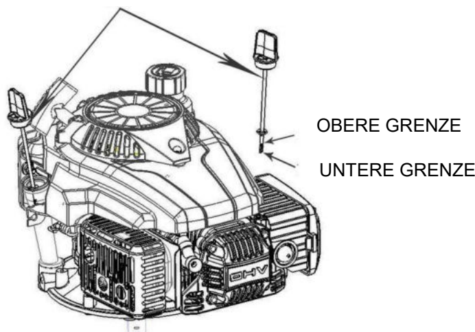
ÖLDECKEL/ÖLMESSTAB
