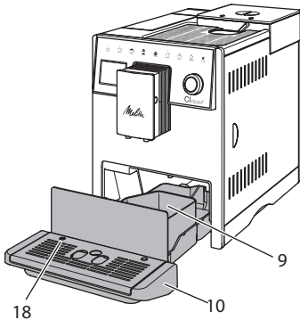
Afb. 10: Lekkakje, residubak en vlotter
