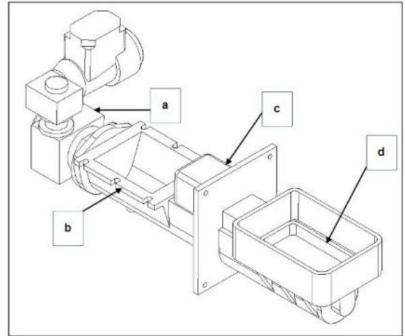
Obr. 2 Konstrukční uspořádání hořáku
