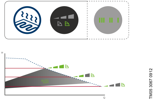
Fig. 25 Sélection du réglage du circulateur en fonction du type d'installation
