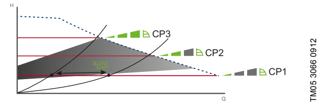
Fig. 26 3 courbes ou réglages à pression constante
