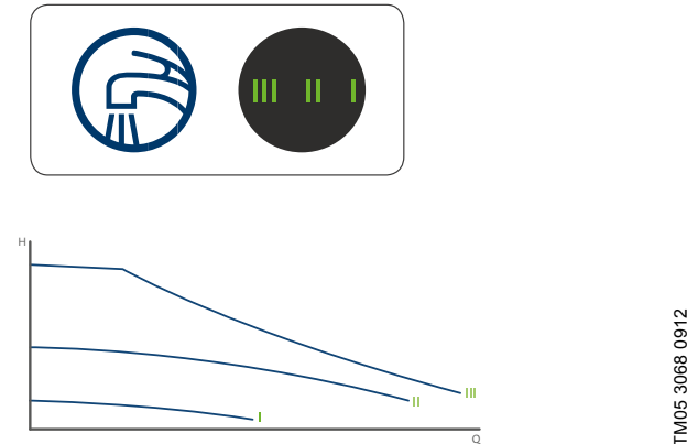
Fig. 27 Sélection du réglage du circulateur en fonction du type d'installation
