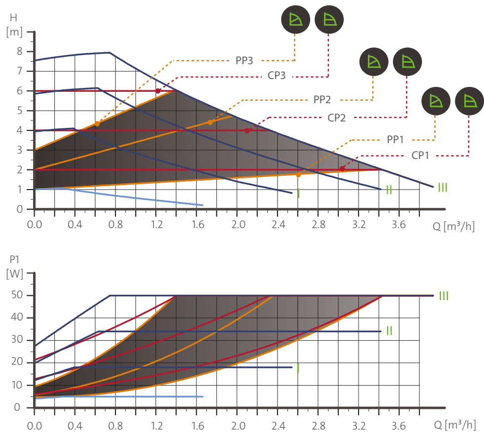
Fig. 42 ALPHA2 et ALPHA3, 25-60 A
