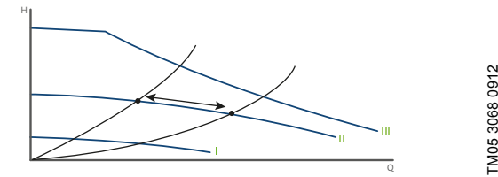
Fig. 28 Trois réglages courbe constante/vitesse constante
