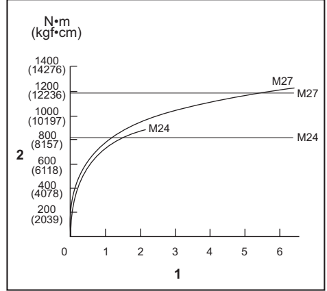
1. Sıkma süresi (saniye) 2. Sıkma torku
