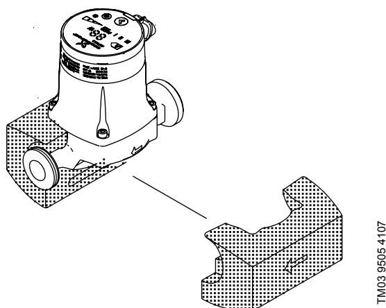
Obr. 18 Tepelně-izolační kryty
