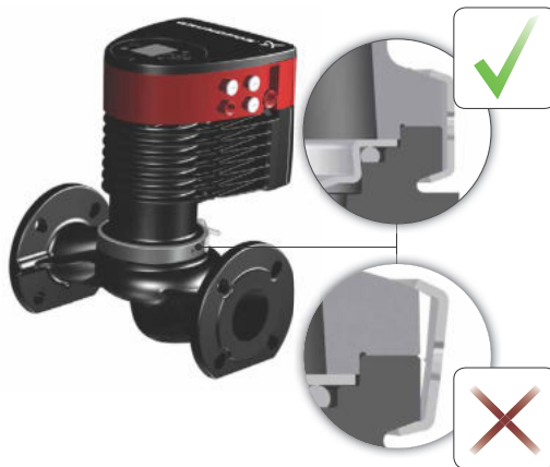
Obr. 13 Upevnění hlavy čerpadla k tělesu čerpadla
