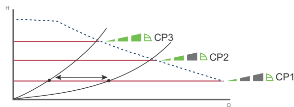
Obr. 24 Tři křivky konstantního tlaku/nastavení
