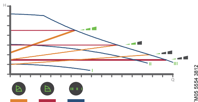
Obr. 22 Volba nastavení čerpadla pro určitý typ soustavy
