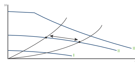
Obr. 25 Tři nastavení s konstantní křivkou
