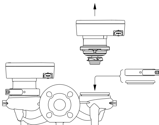
Obr. 29 Poloha zaslepovací přírubby
