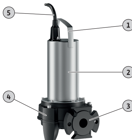
Fig. 1: Áttekintés
