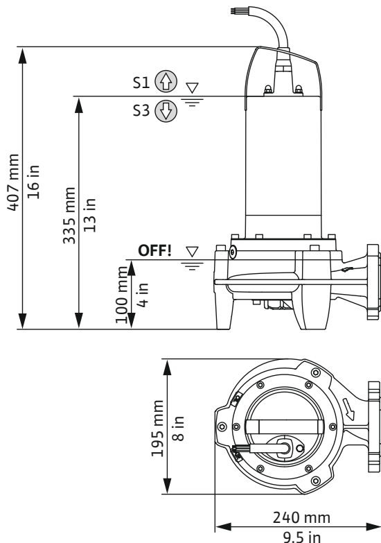
Fig. 3: Telepítési méretek
