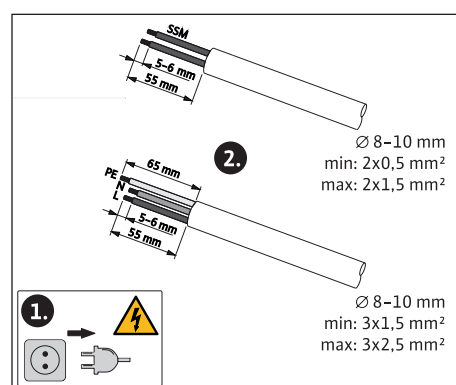
Ábra 15: A csatlakoztatás előkészítése
