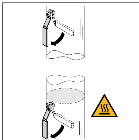
Ábra 12: Az elzárószerelvények nyitása
