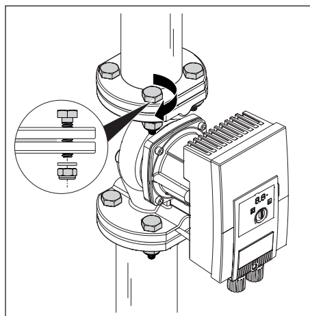
Ábra 8: A szivattyú szerelése
