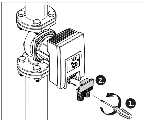
Ábra 16: A dugasz leszerelése
