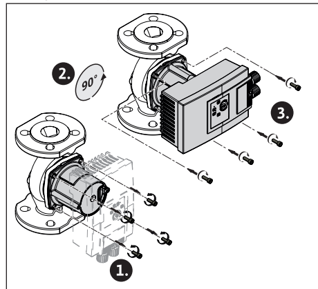
Ábra 5: A motor igazítása
