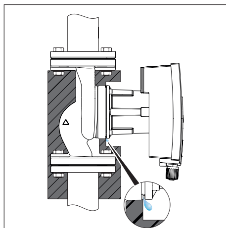
Ábra 13: Szigetelés, a kondenzátumlefolyó szabadon hagyása
