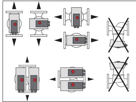
Ábra 4: Megengedett beépítési helyzetek
