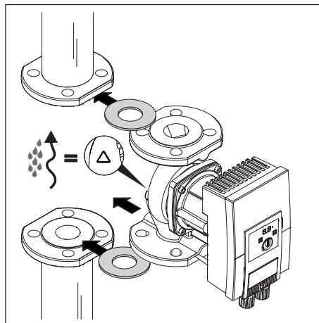
Ábra 7: A szivattyú behelyezése
