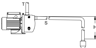
Obr. 1 Potrubní přípojka
