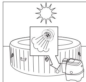
Vzduch expanduje v poledne. Tlakový odvězdušňovací ventil se aktivuje a uvolní přebytečný vzduch.
