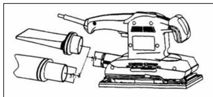
Obr. 2 - Připojení odsávacího prachu
