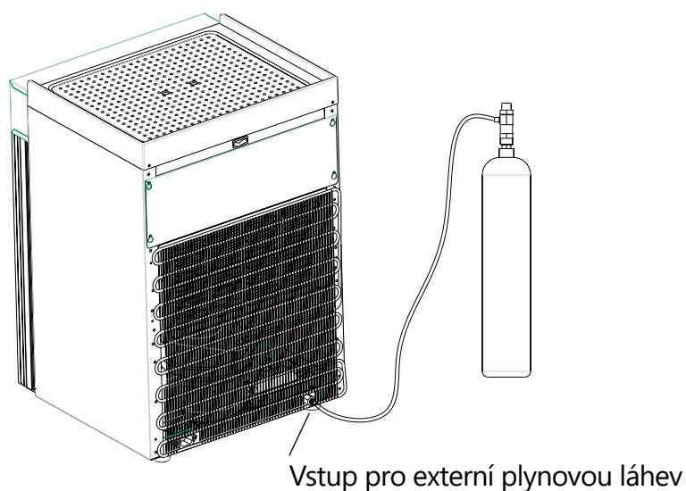
Obrázek jednokomorového systému na 4 láhve - VT4
