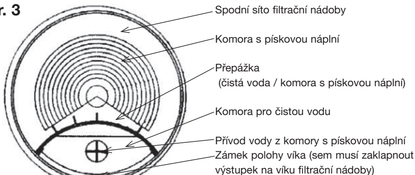
Pohled na filtrační nádobu bez víka
