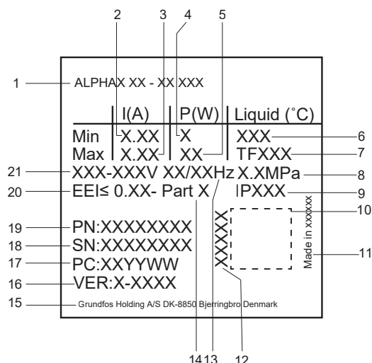
Tabliczka znamionowa
